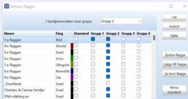
Bild 4. Redigera flaggor.
