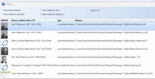
Bild 1. Byrålådan.
