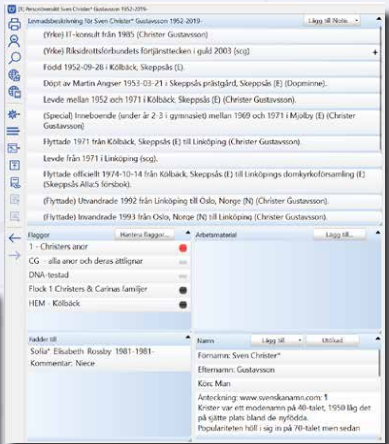
Bild 2. Egen panellayout.
